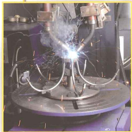
Saldatura a filo continuo automatica Automatic seam-welding
