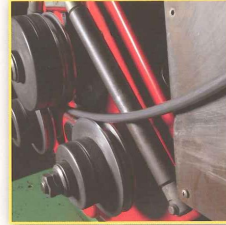
Calandratura tubi Pipes calendaring
