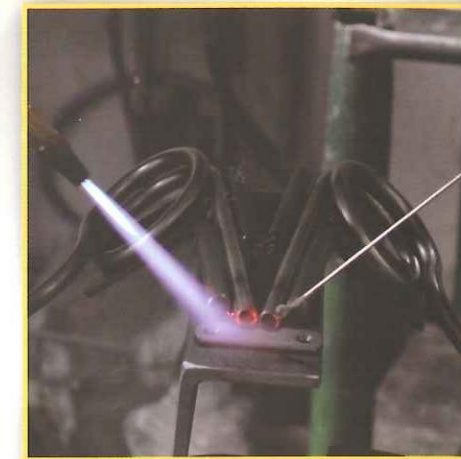
Saldatura ad argento Silver welding
